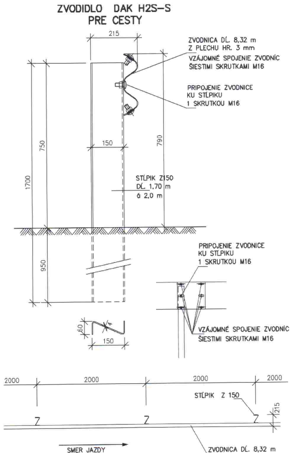
Obrázok 23 – Zvodidlo DAK H2S-S v (mm)
