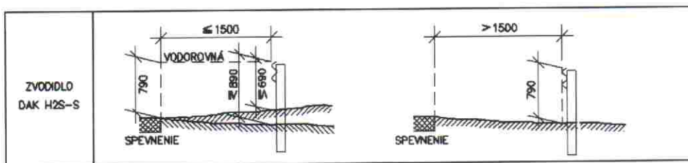
Obrázok 7.1 – Výška jednostranných zvodidiel (mm)
