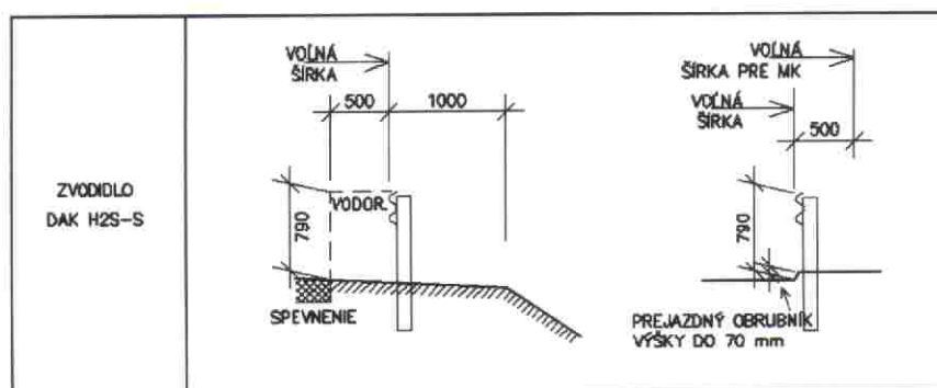
Obrázok 9.1 – Jednostranné zvodidlá na krajnici (mm)
