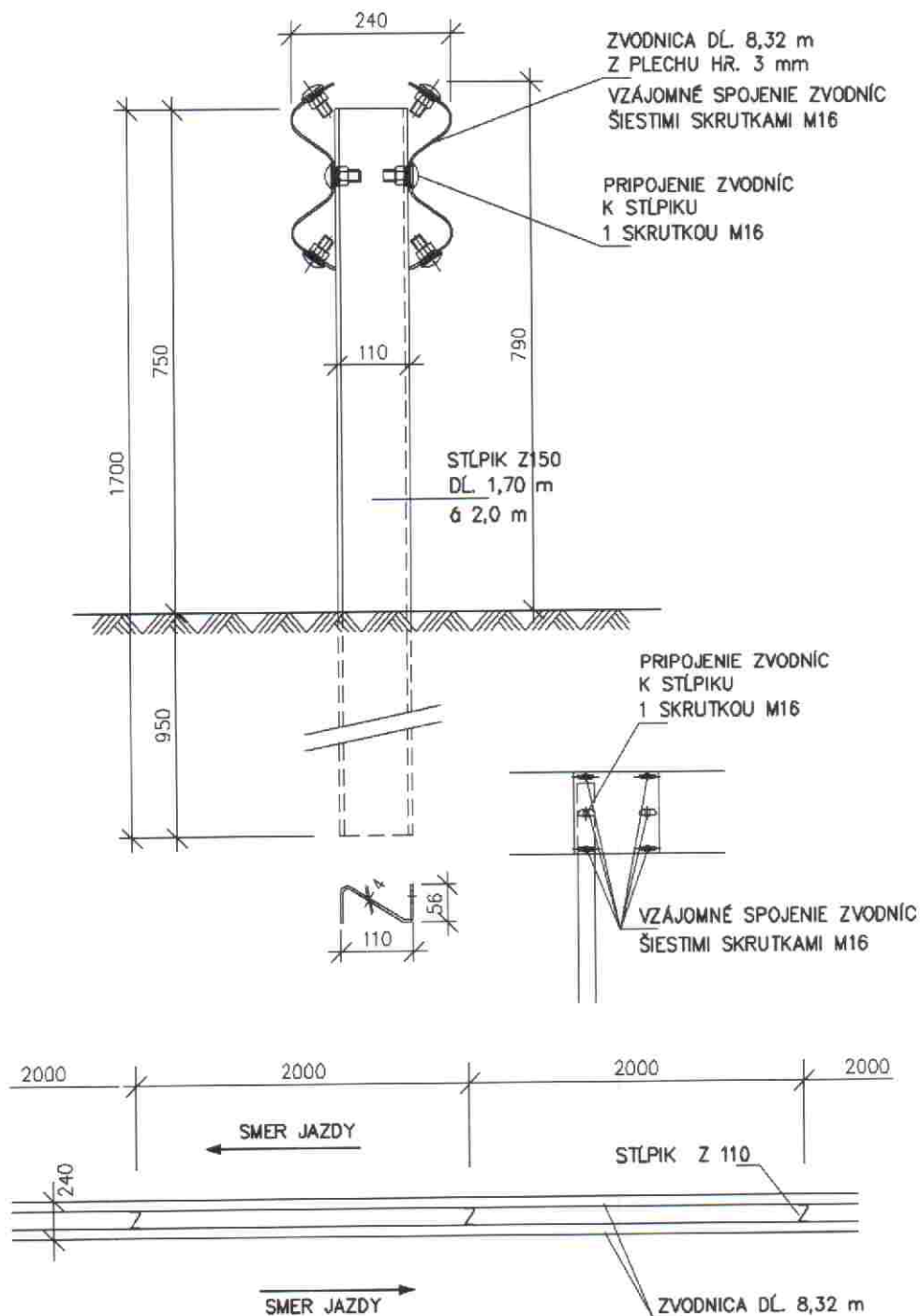
Obrázok 24 – Zvodidlo DAK H2D-S v (mm)
