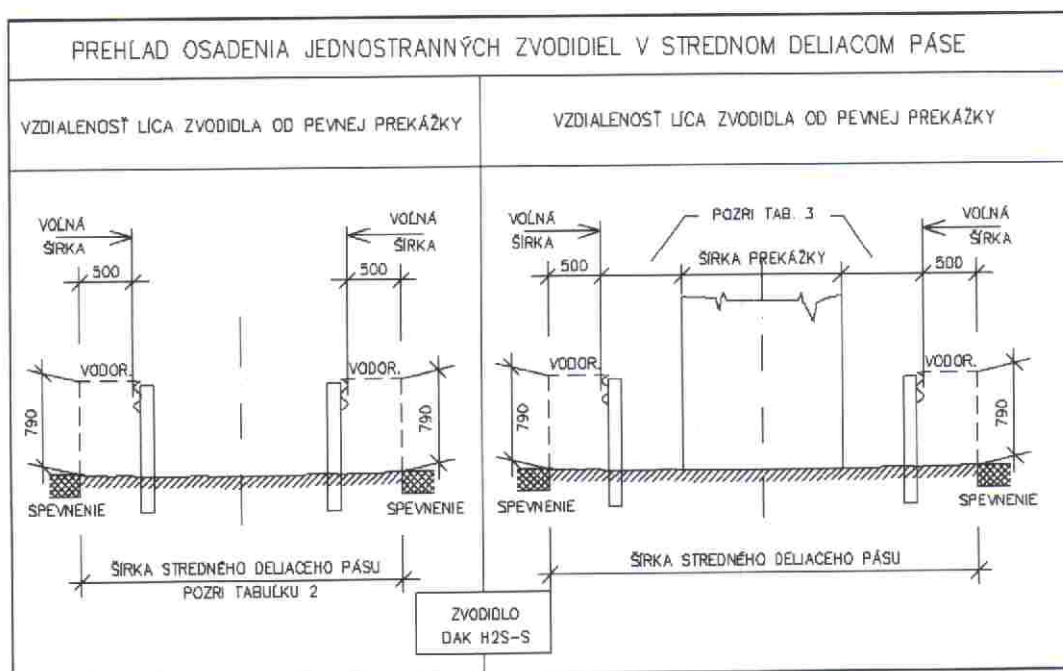
Obrázok 10.1 – Jednostranné zvodidlá v strednom deliacom páse (mm)
