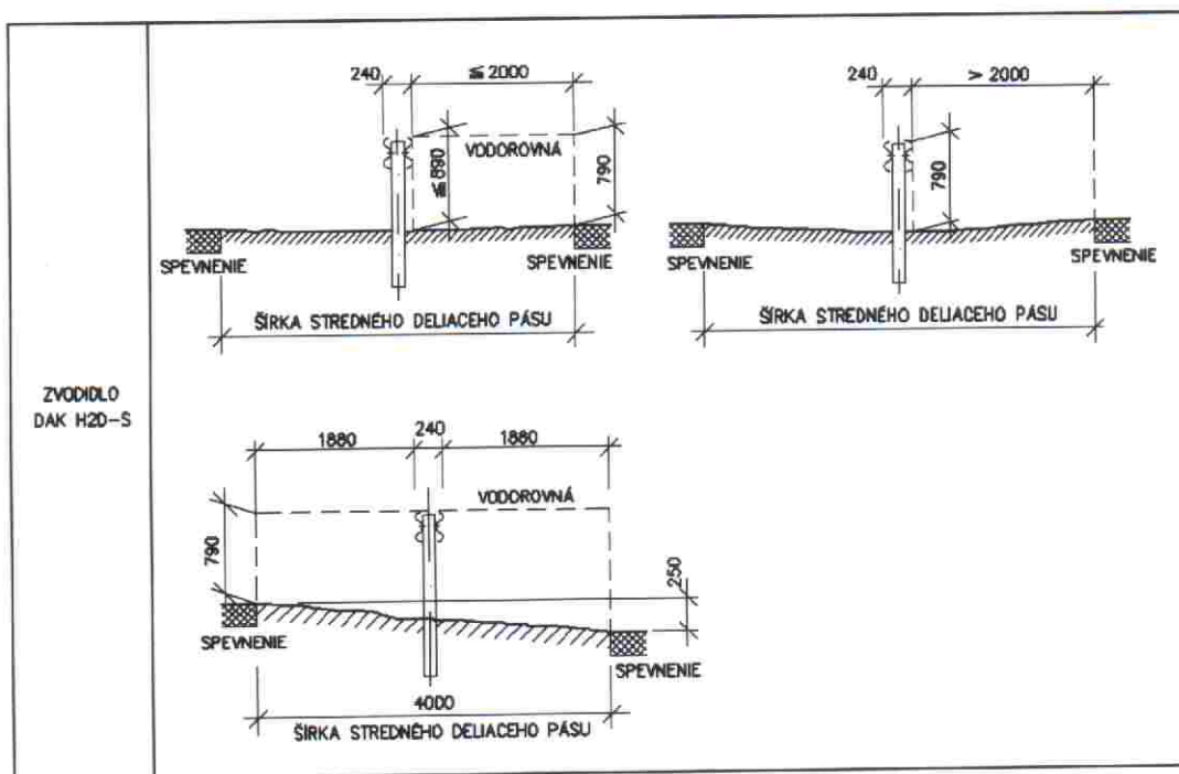
Obrázok 8.1 – Výška obojstranných zvodidiel (mm)
